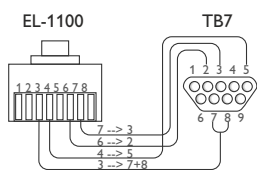
Схема подключения дата-кабеля
